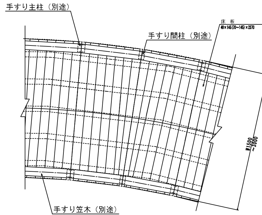
床伏せ図 (詳細図)
